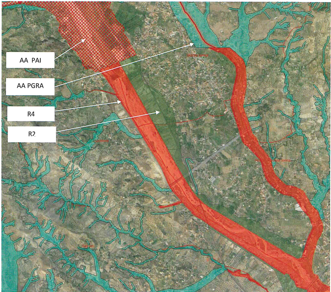
Piano Stralcio di Assetto idrogeologico dell'ex ABR Calabria - rischio idraulico Comune di Grotteria (RC) – fiumara Torbido - proposta di ripermimetrazione
