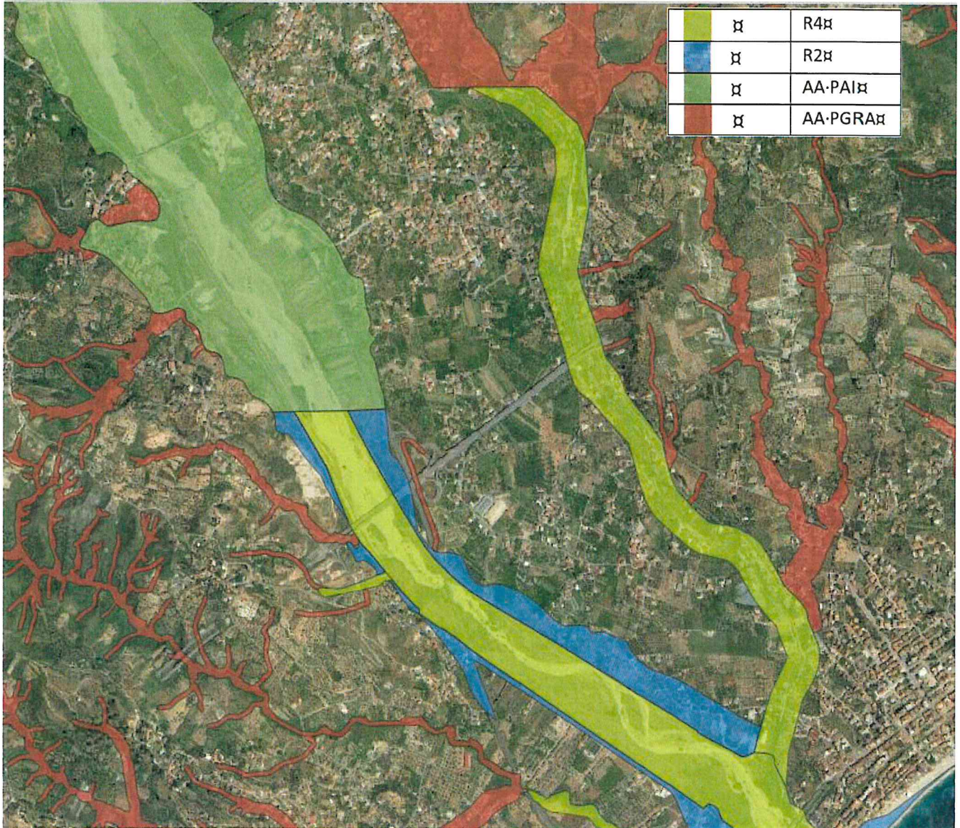
Piano Stralcio di Assetto idrogeologico dell'ex ABR Calabria - rischio idraulico Comune di Grotteria (RC) – fumara Torbido -Piano Vigente
